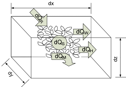
Şekil 4. Bitki elemanları için enerji dengesi.
