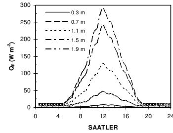
Şekil 8. Bitki standında net radyasyon değişimi
