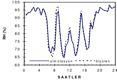
Şekil 20. Bitki standında ölçülen ve hesaplanan bağıl nem
